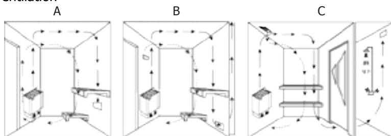
Рис. 7 Вентиляция в сауне Fig. 7 Air ventilation
