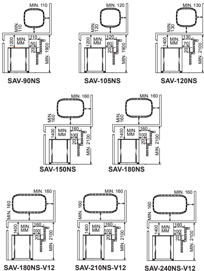
Abb 2 | Mindest Sicherheitsabstände (mm) Fig. 2 | Minimum safety distances (mm)
