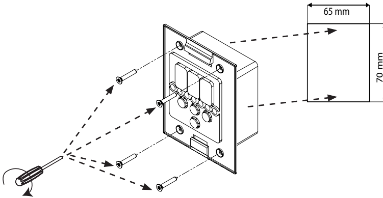
afb. 5 Montage bedieningspaneel Pro D
