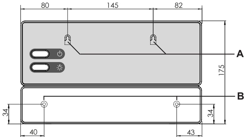
Bild 2 Position på upphängningsanordningen och monteringshålen (mått i mm)
