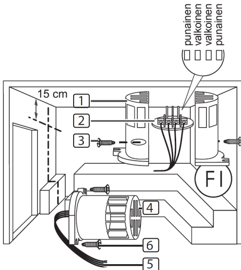
Kuva 8 Kiuasanturin asentaminen
