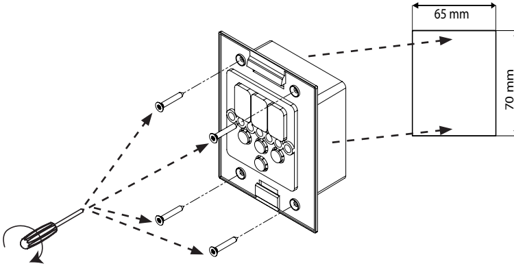
Kuva 5 Pro D -hallintalaitteen asennus
