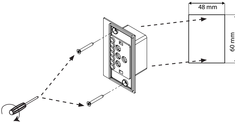
Kuva 6 Hallintalaitteen lisälähdön asennus (valinnainen)
