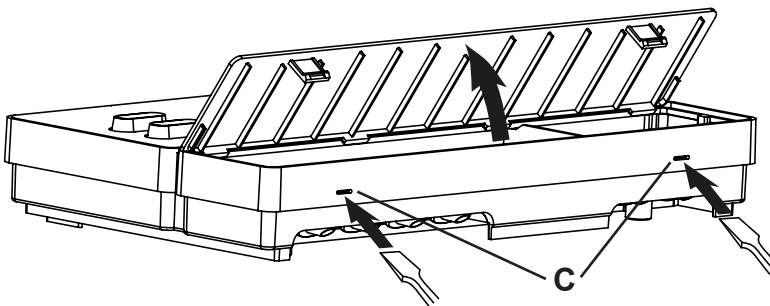
afb. 3 Behuizingsdeksel verwijderen
